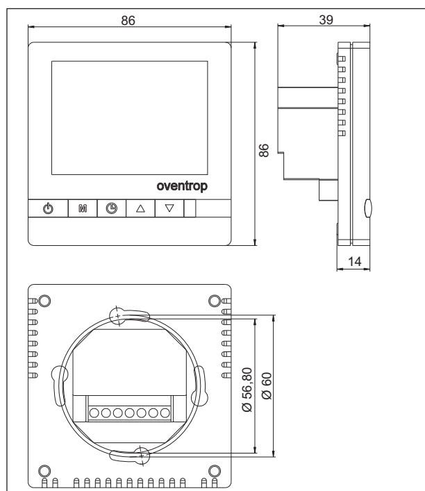
Размеры
