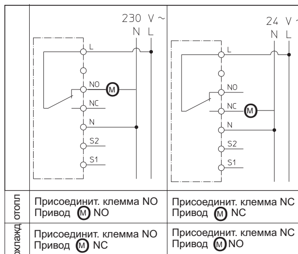
Схема подключения
